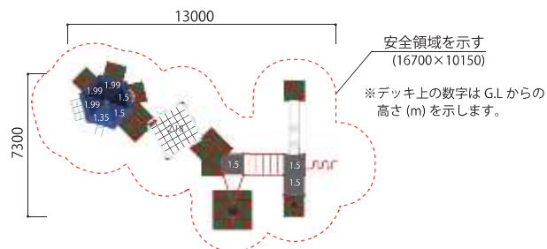
平面図 Scale=1:200
